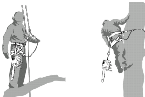
Fig. 3 – Esempi di attacchi della motosega all'imbracatura dell'operatore
